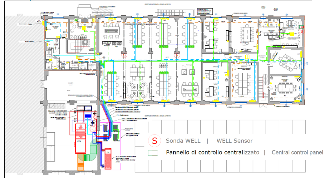
Piano terra - Impianto di climatizzazione - scala 1:100
