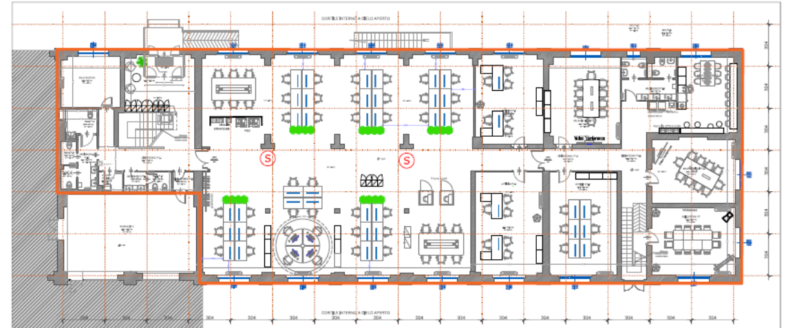
PIANTA PIANO TERRA _ ARREDI STATO DI PROGETTO _ SCALA 1:100 GROUND FLOOR PLAN _ FURNISHINGS STATE OF PROJECT _ SCALE 1:100
