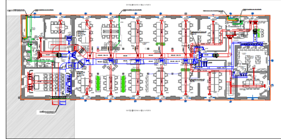
Piano terra - Impianto di ventilazione - scala 1:100
