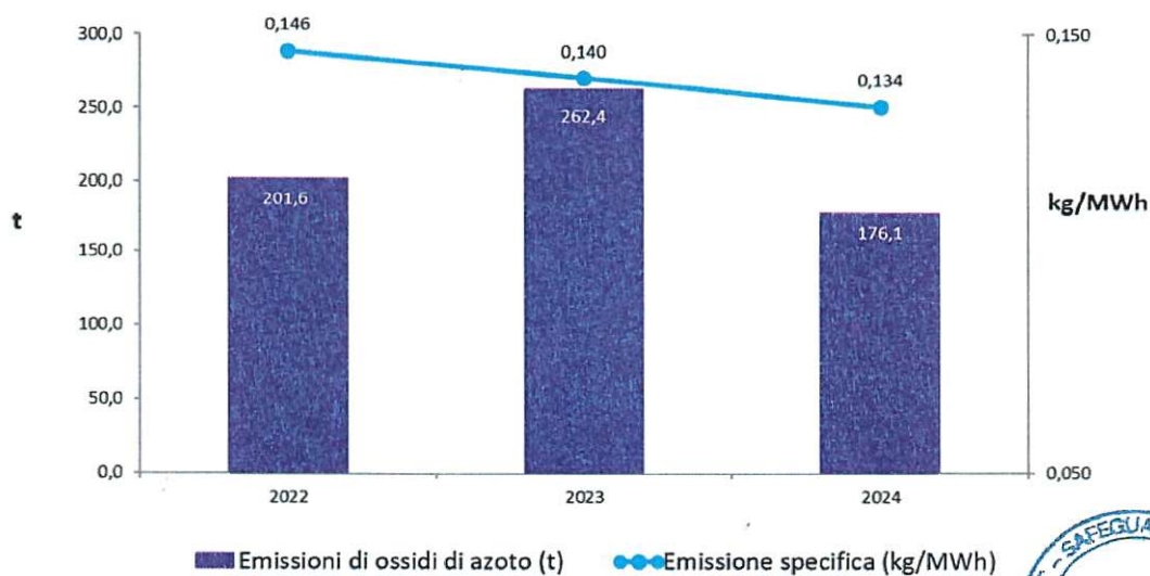
Grafico 4 - Emissioni quantitative di NOx
