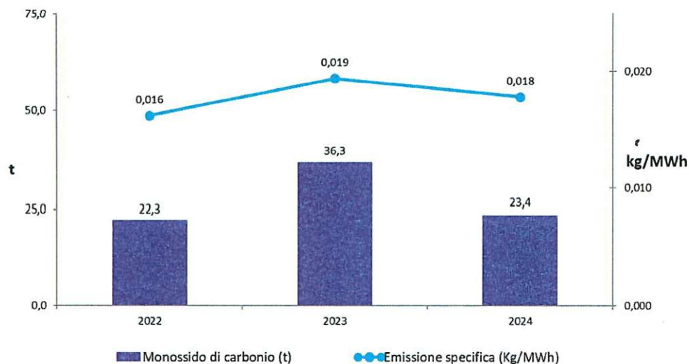
Grafico 5 - Emissioni quantitative di CO
