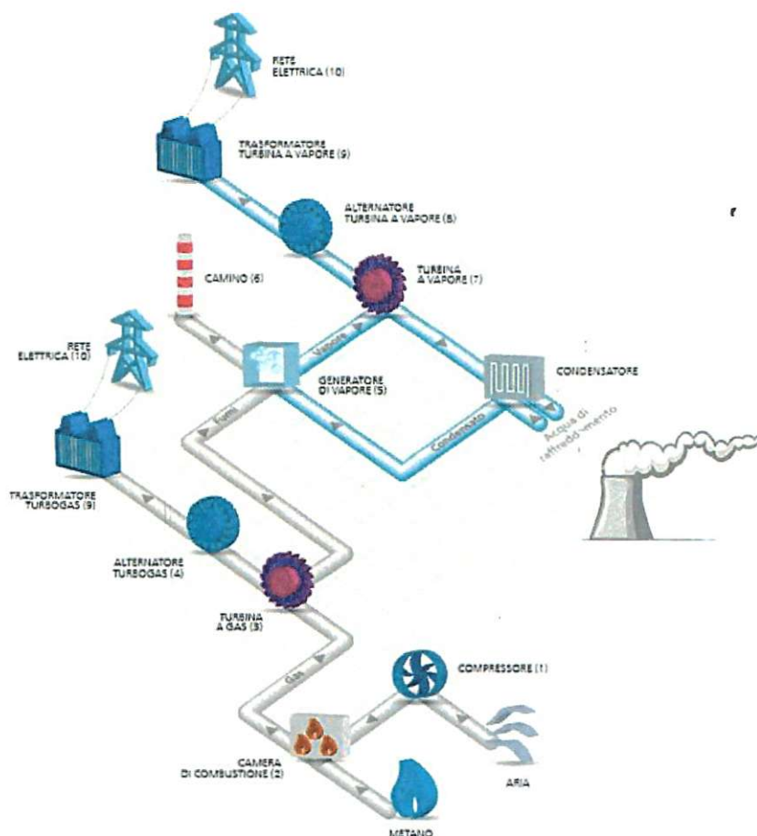
Figura 6 - Schema di principio del ciclo combinato
