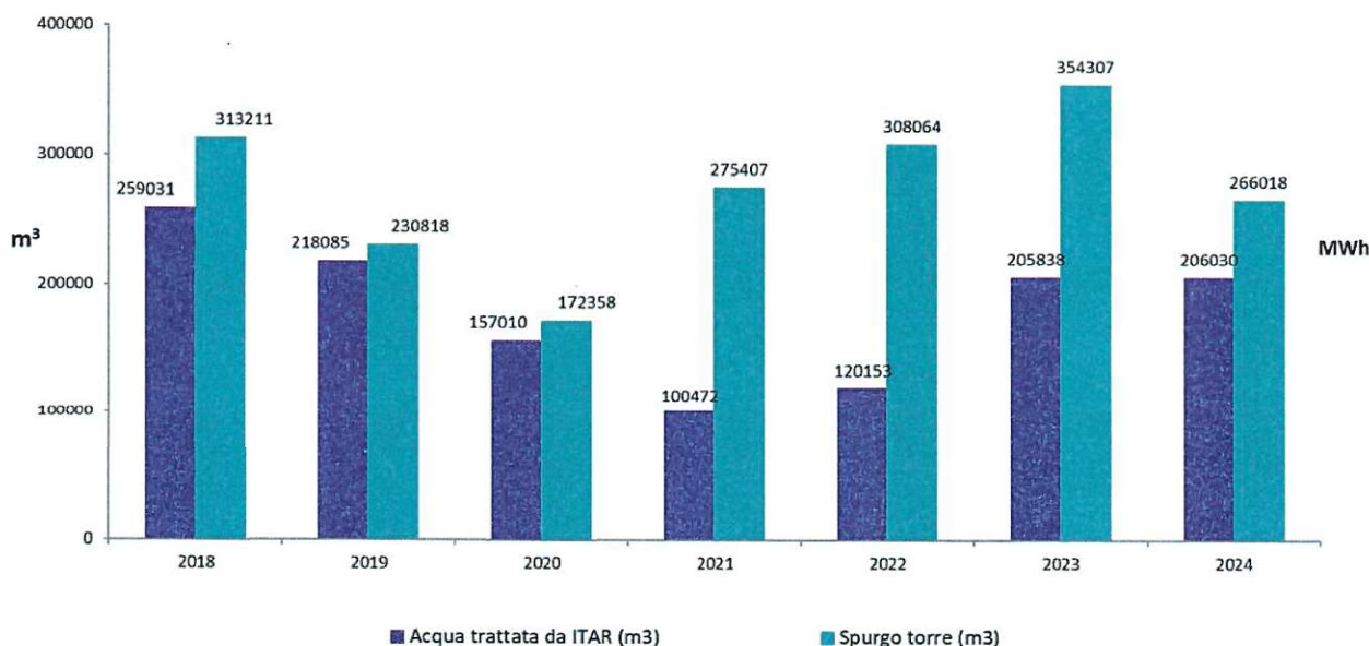
Grafico 7 - Ripartizione dei quantitativi delle acque reflue
