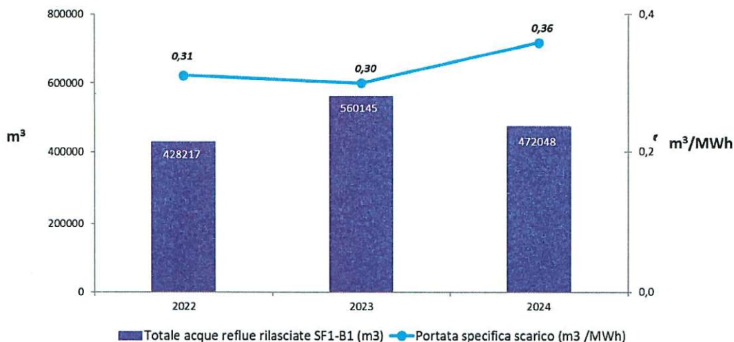
Grafico 6 - Quantitativi di acque reflue scaricate
