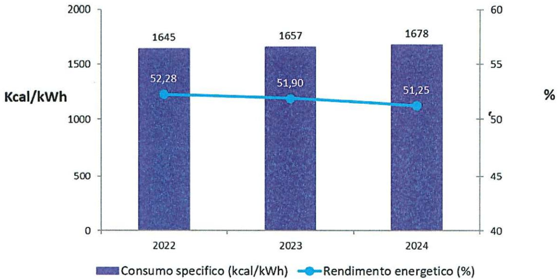
Grafico 13 - Andamento consumo specifico e rendimento energetico
