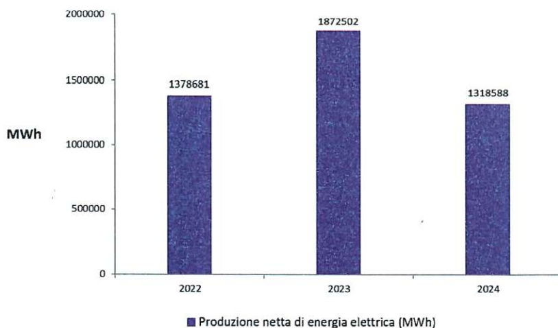
Grafico 2 - Andamento della produzione in ciclo combinato
