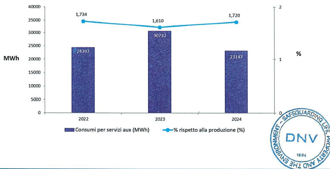
Grafico 12 - Indicatore di efficienza energetica dell'impianto
