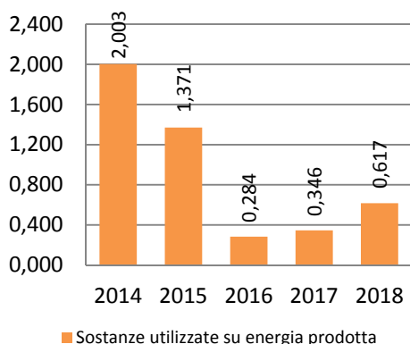
Grafico 9 – Sostanze utilizzate riferite all'unità di energia prodotta (dati in t/GWh)
