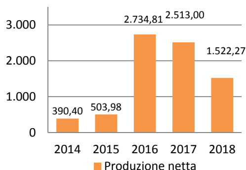
Grafico 1 – Produzione netta di energia elettrica (dati in GWh)
