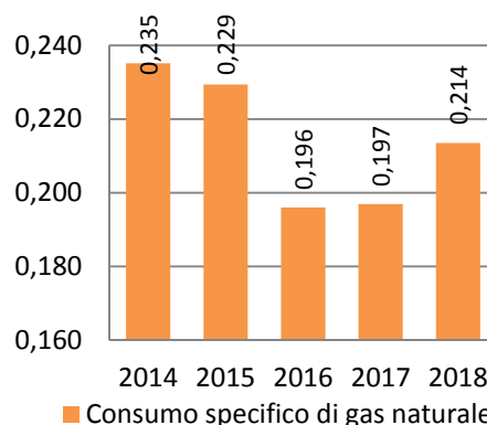
Grafico 11 – Consumo specifico di gas naturale (dati in milioni di Sm 3 /GWh)
