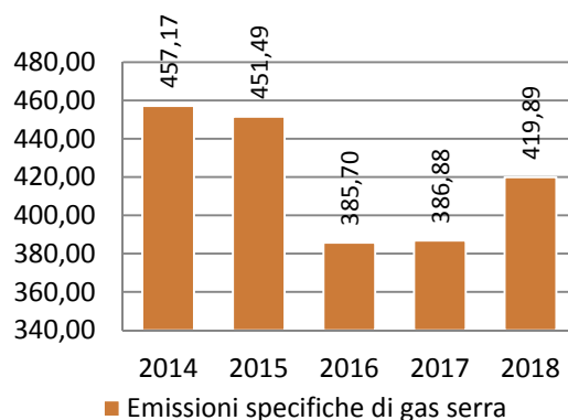
Grafico 5 – Emissioni specifiche di gas serra espresse come CO 2 equivalente (dati in t/GWh netti prodotti)
