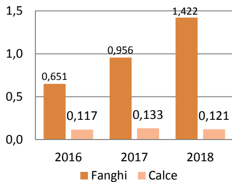
Grafico 8 – Produzione fanghi per refluo prodotto ITAR e utilizzo calce riferiti alla somma della quantità di refluo prodotto ITAR e produzione acqua industriale (dati in Kg/m 3 )
