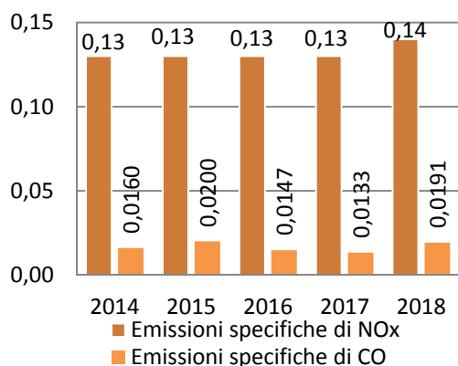
Grafico 2 – Emissioni specifiche di NO x e CO (dati in t/GWh netti prodotti)
