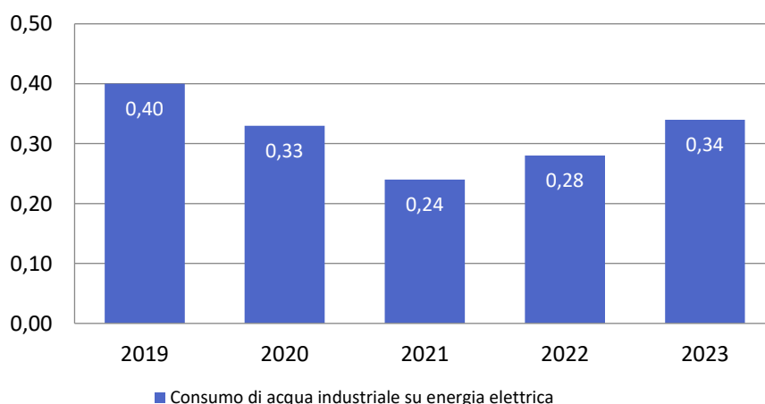
Grafico 15 – Consumo specifico di acqua industriale (dati in m 3 /MWh)
