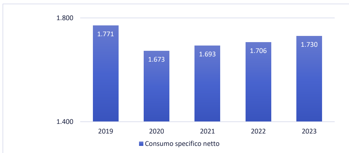
Grafico 12 – Consumo specifico netto vettore gas naturale (dati in kcal/kWh)
