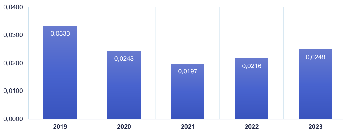
Grafico 14 – Consumo specifico di energia elettrica per servizi ausiliari (dati in kWh/kWh)
