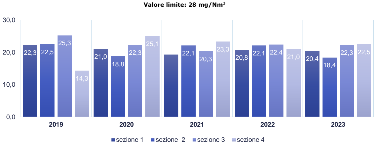
Grafico 3 – Concentrazioni medie annue di NO x rilevate nei fumi emessi (valori riferiti a gas normalizzati secchi riportati a un tenore di ossigeno pari al 15% ed espressi in mg/Nm 3 )
