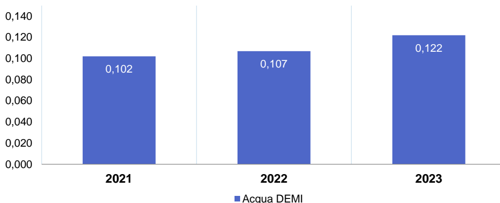
Grafico 9 – Indicatore specifico di prestazione: Acqua DEMI/Energia prod netta (dati in m 3 /MWh)
