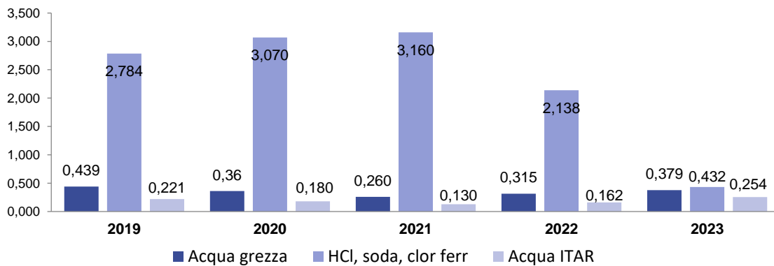
Grafico 8 – Indicatori specifici di prestazione: acqua grezza/Energia prod netta (dati in m 3 /MWh) - HCl soda clor ferr/acqua demi prodotta (dati in kg/m 3 ) - Acqua itar/Energia prod netta (dati in m 3 /MWh)
