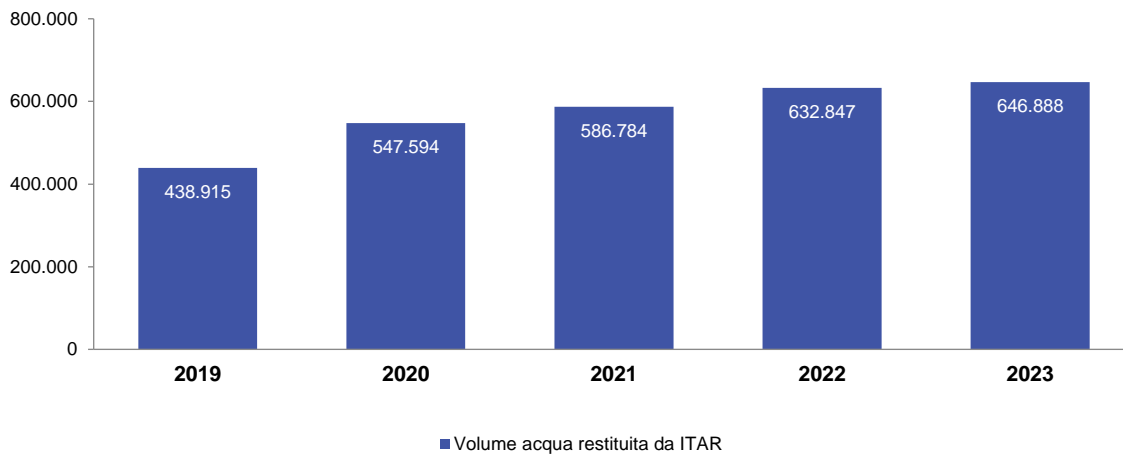
Grafico 6 – Volume complessivo acqua restituita da impianto ITAR (dati in m 3 )
