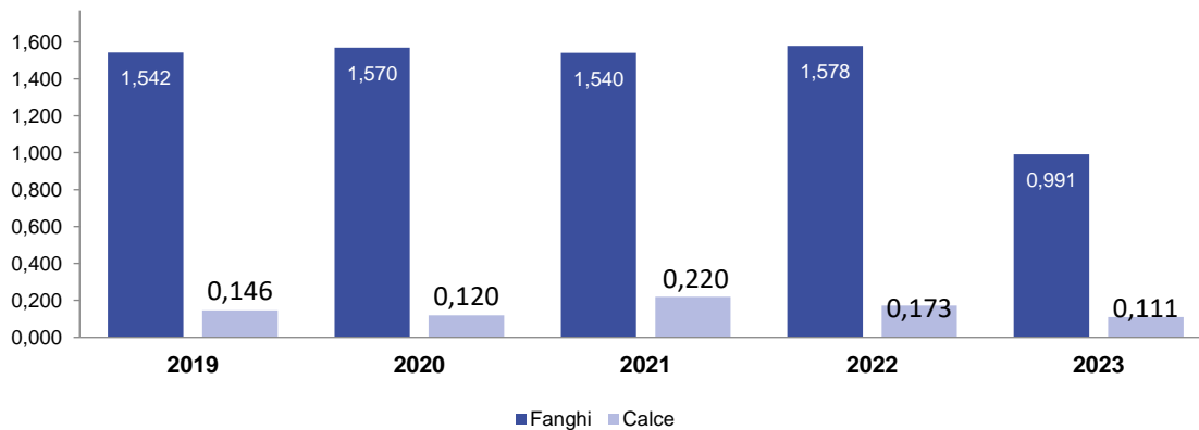
Grafico 7 – Produzione fanghi per refluo prodotto ITAR ed utilizzo di calce riferito alla somma della quantità di refluo prodotto ITAR e produzione acqua industriale (dati in kg/m 3 )
