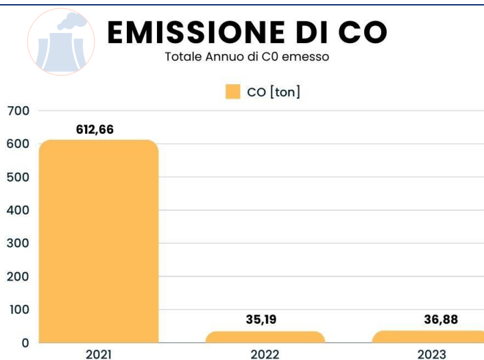
Grafico 4 – Emissione di CO e relativo indicatore
