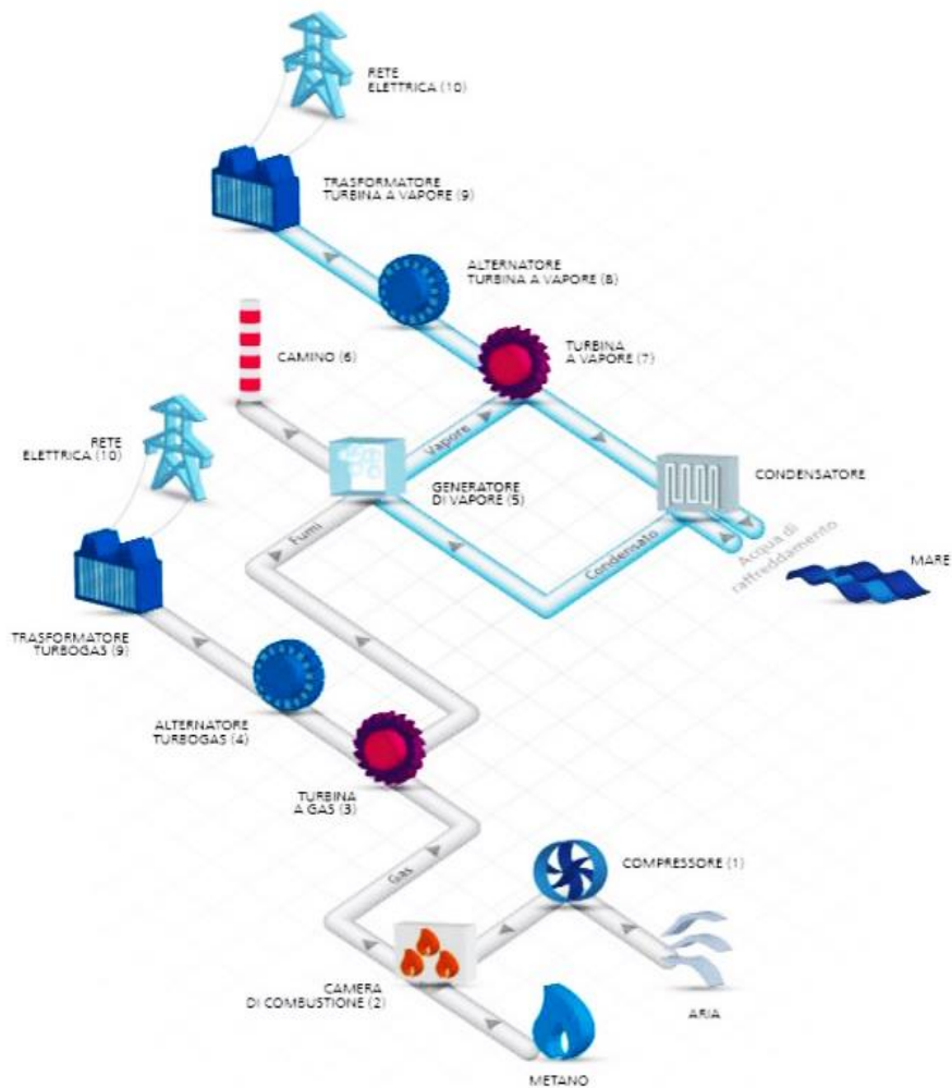
Figura 6 - Schema di processo di una centrale Termoelettrica a ciclo combinato
